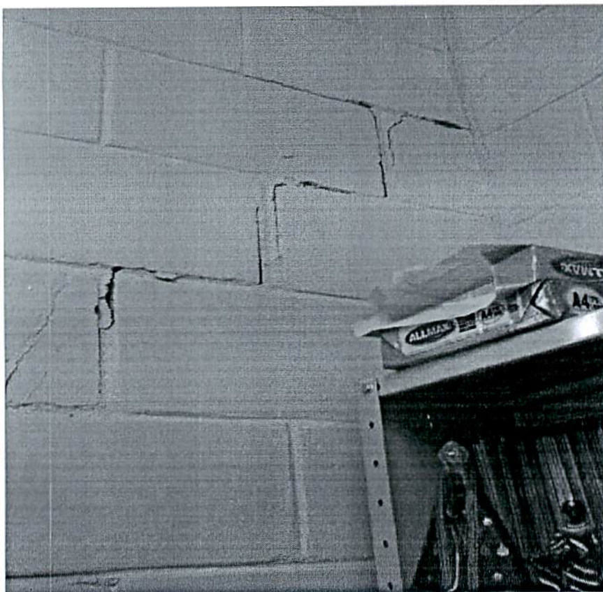
Rachadura em parede da Escola Estadual (Foto 003)
