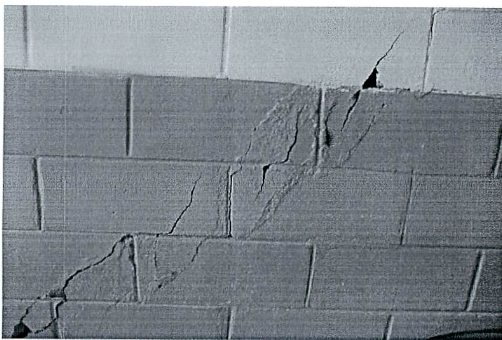
Rachadura em parede da Escola Estadual (Foto 002)
