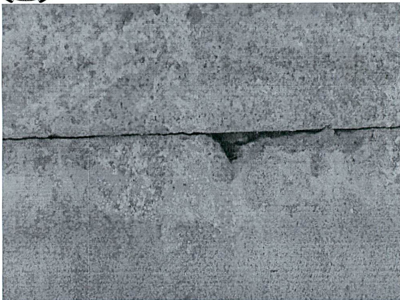
Piso sem desenpenação da quadra poliesportiva da Escola Estadual (Foto 005)
