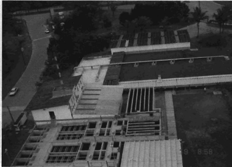
Figura 13 – Estação de Tratamento de Água da Riviera de São Lourenço
